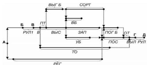
Рис. 1. Модельный технологический график наземного обслуживания ВС
